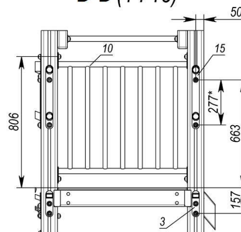
B-B (1 : 15)
