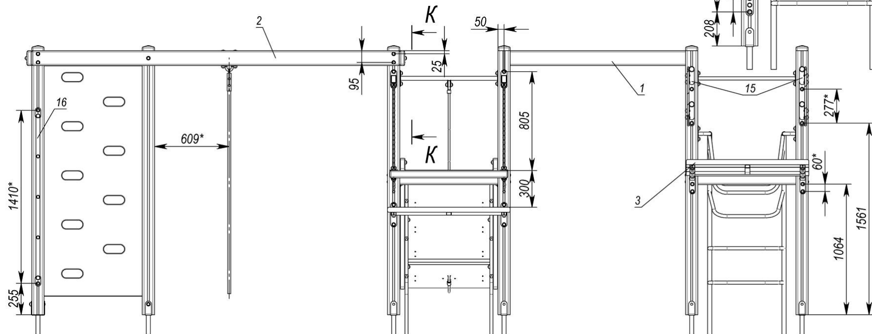
G-G (1 : 20)
