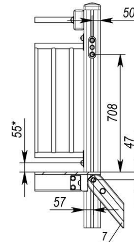
E-E (1 : 15)
