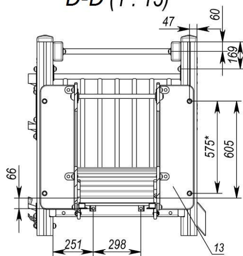
D-D (1 : 15)
