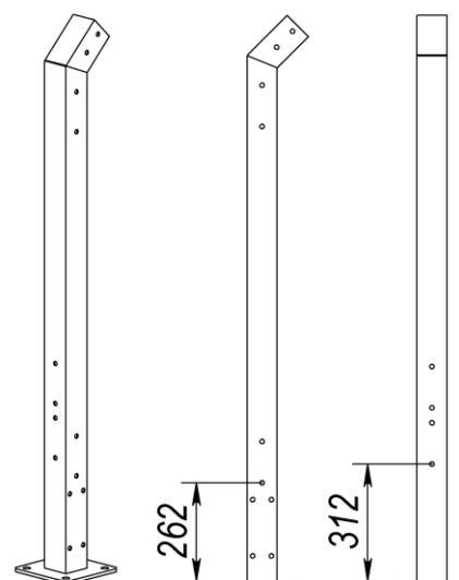
Corner column №2
