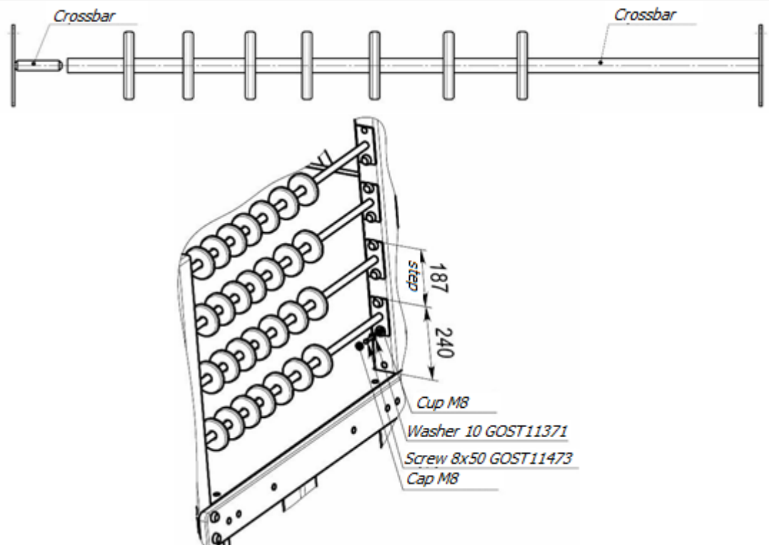
Picture 24 «Counting frame fastening»
