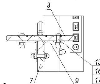
B-B (1 : 4)
