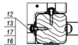
В-В (1 : 5)
