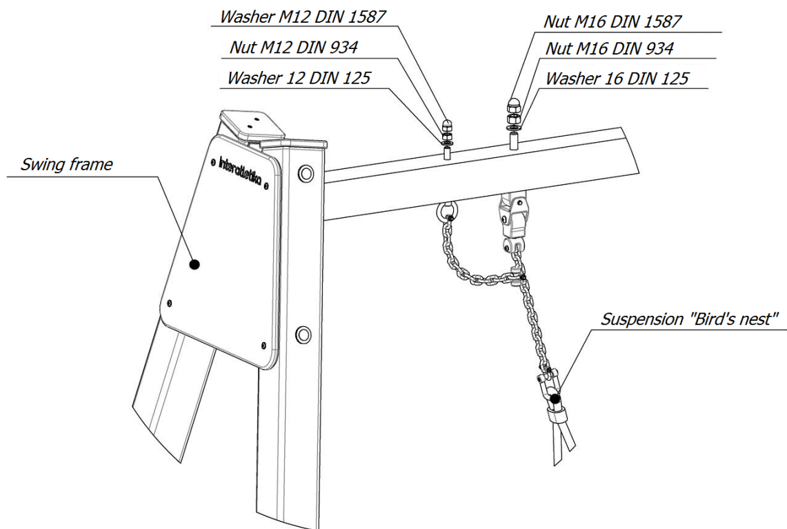
Picture 2 – Fixing scheme of «Bird's Nest»
