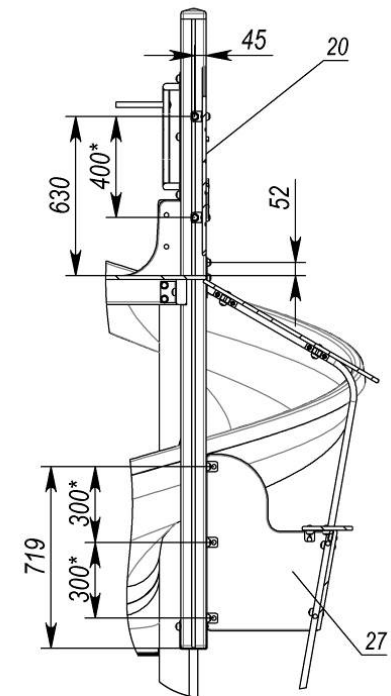
M-M (1 : 20)
