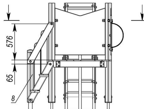
L-L (1 : 25)
