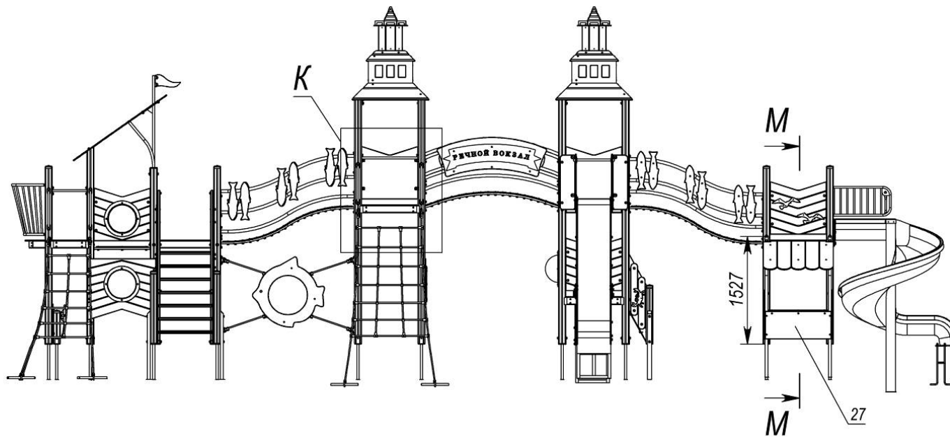
I (1 : 50)
