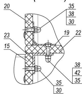
A-A (1 : 2.5)
