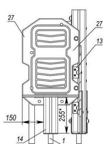
B-B (1 : 10)
