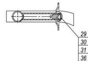
A-A (1 : 4)
