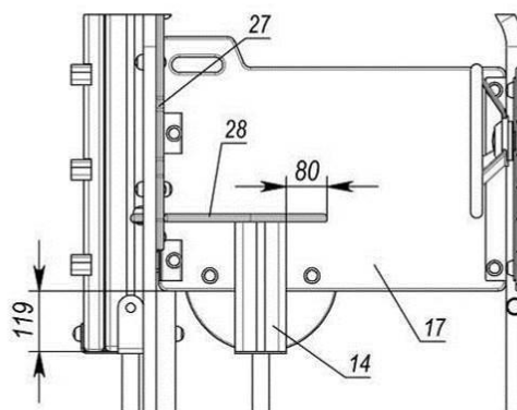
C-C (1 : 10)
