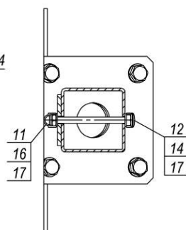
B-B (1 : 5)
