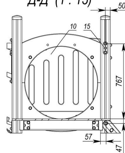
Д-Д (1 : 15)
