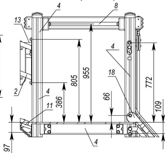
В-В (1 : 15)
