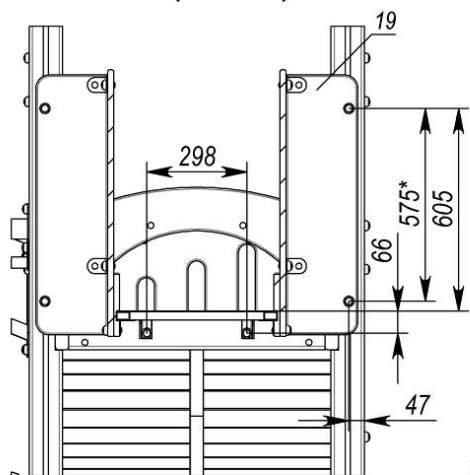
Г-Г (1 : 15)
